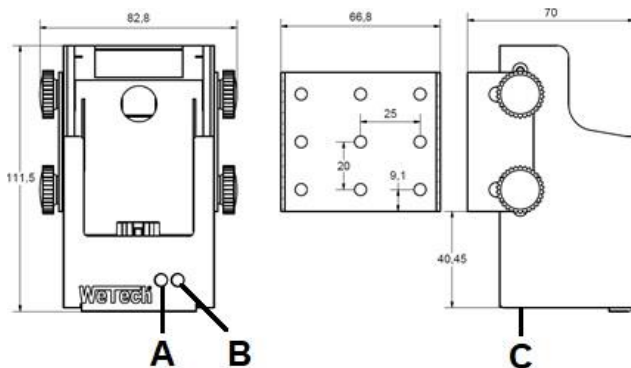
Schemazeichnung WTC669
